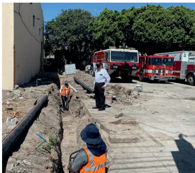
Se ejecutaron trabajos de introducción de drenaje sanitario en el inmueble del Heroico Cuerpo de Bomberos de Ciudad Fernández.
